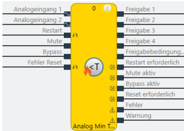
Abb. 193: Logische Anschlüsse für den Funktionsblock Analog Min Temperatur
