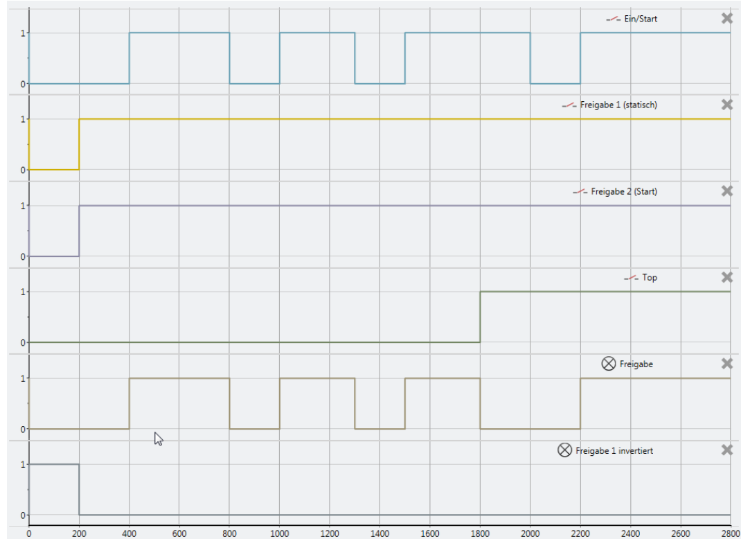
Abb. 148: Typisches Ablauf-/Timingdiagramm für den Funktionsblock Presse Einrichten
