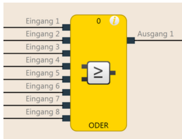
Abb. 50: Funktionsblockdiagramm für den Funktionsblock ODER
