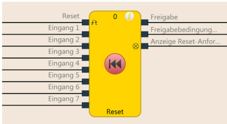
Abb. 78: Funktionsblockdiagramm für den Funktionsblock Reset
