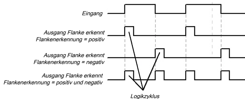
Abb. 68: Timingdiagramm für den Funktionsblock Flankenerkennung
