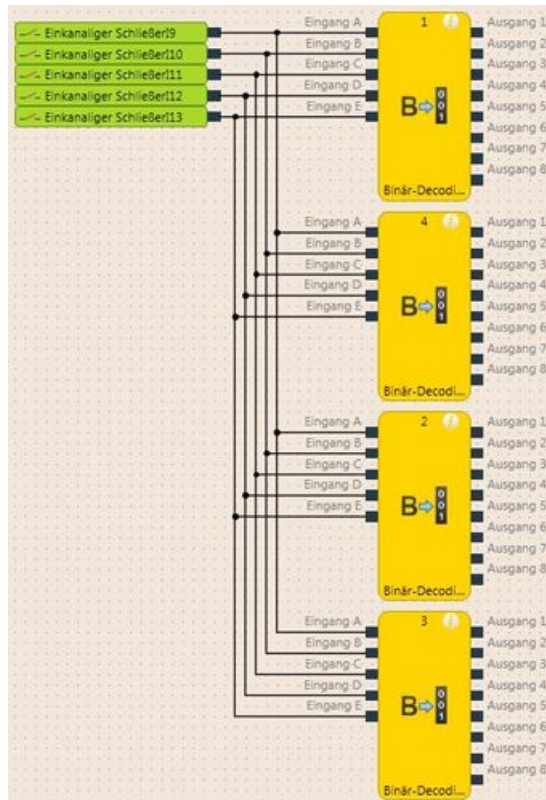
Abb. 71: Kombination von vier Binär-Decodierern
