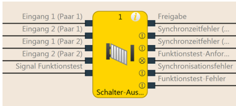
Abb. 109: Funktionsblockdiagramm für den Funktionsblock Schalter-Auswertung
