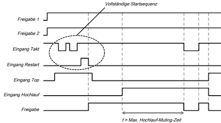
Abb. 164: Ablauf-/ Timingdiagramm, wenn der Eingang Takt Low, maximale Hochlauf-Muting-Zeit > 0 und Wiederanlauf-sperre auf 3 - Nach Stillstand im Abwärtshub oder Ausgangsstellung gesetzt ist.
