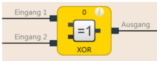
Abb. 51: Funktionsblockdiagramm für den Funktionsblock XOR (exklusives ODER)
