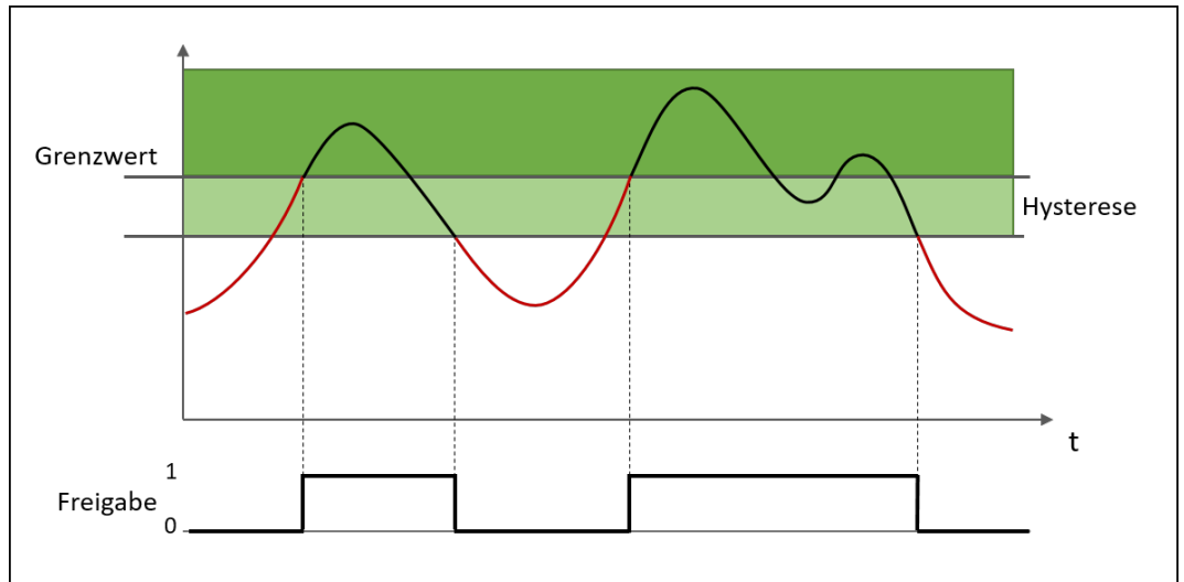
Abb. 186: Überwachung auf "Unterschreitung"
