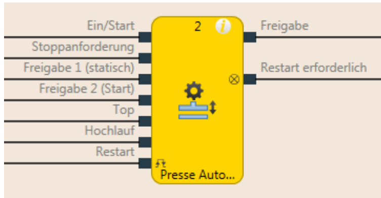
Abb. 155: Logische Anschlüsse für den Funktionsblock Presse Automatik
