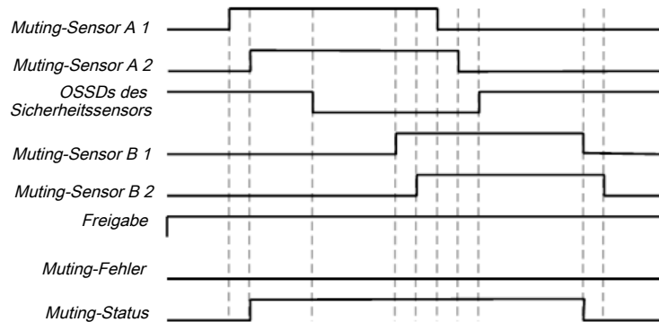
Abb. 122: Gültige Muting-Sequenz bei Benutzung der Konfigurations-Grundeinstellung
