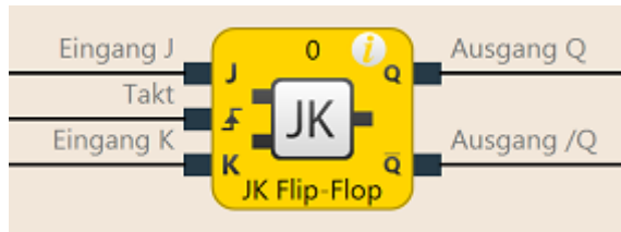
Abb. 54: Logische Anschlüsse für den Funktionsblock JK Flip-Flop
