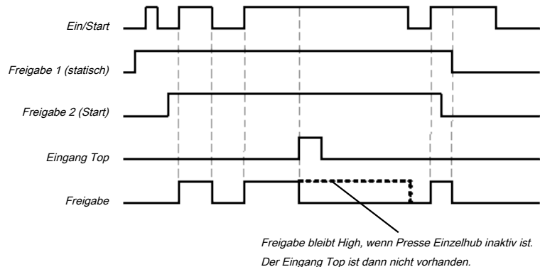
Abb. 149: Ablauf-/ Timingdiagramm für den Funktionsblock Presse Einrichten
