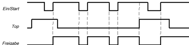
Abb. 153: Ablauf-/ Timingdiagramm für den Funktionsblock Presse Einzelhub bei Konfiguration von Ein/Start auf 1 - Tippen
