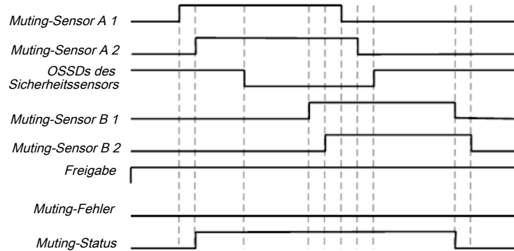
Abb. 125: Gültige Muting-Sequenz bei Benutzung der Konfigurations-Grundeinstellung
