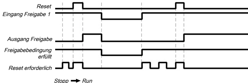
Abb. 205: Ablauf-/Timing-Diagramm für den Funktionsblock
