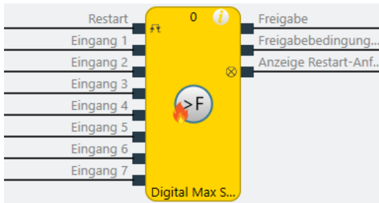
Abb. 210: Logische Anschlüsse für den Funktionsblock Digital Max Strömung
