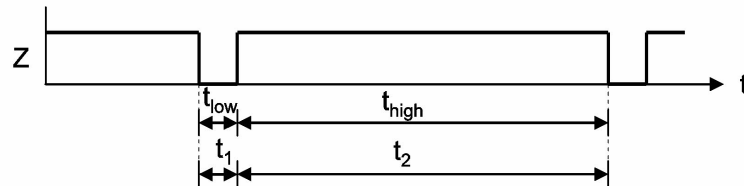
Abb. 101: Signalmuster für einzelnes Pulsgebersignal
