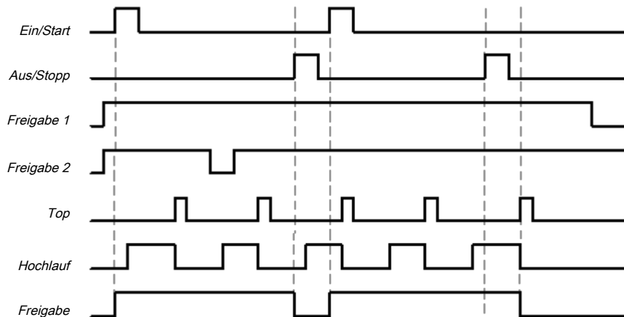
Abb. 156: Typisches Ablauf-/Timingdiagramm für den Funktionsblock Presse Automatik
