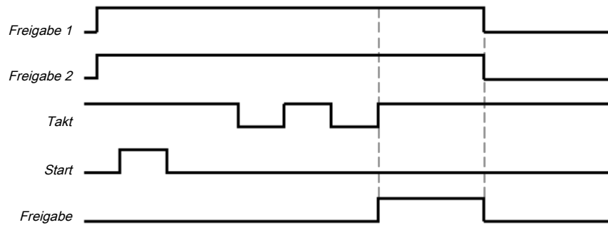
Abb. 160: Ablauf-/ Timingdiagramm für eine vollständige Startsequenz im Schweden-Modus im Zweitaktbetrieb
