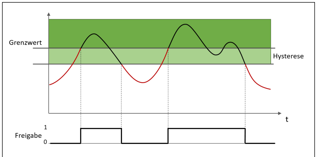
Abb. 198: Überwachung auf "Unterschreitung"
