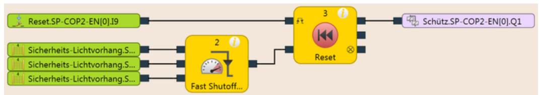
Abb. 61: Konfigurationsbeispiel für Fast Shut Off mit drei Lichtvorhängen
