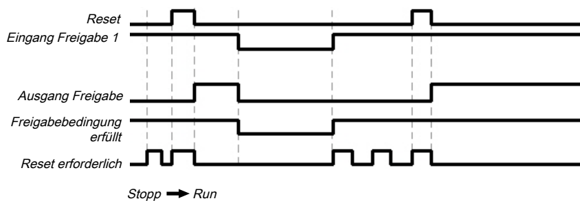
Abb. 217: Ablauf-/Timing-Diagramm für den Funktionsblock
