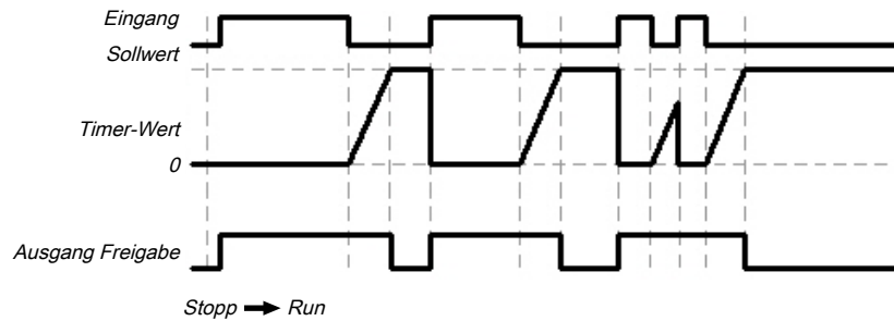
Abb. 83: Ablauf-/Timingdiagramm für den Funktionsblock Abschaltverzögerung
