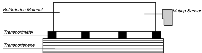
Abb. 118: Erkennen von Material beim Muting
