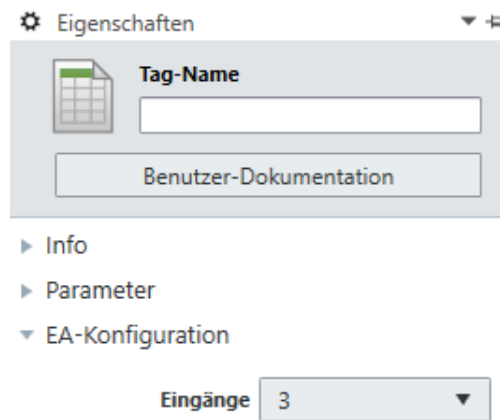
Abb. 74: E/A-Konfiguration für den Funktionsblock Log-Generator
