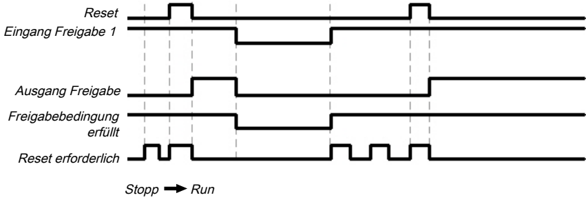
Abb. 221: Ablauf-/Timing-Diagramm für den Funktionsblock
