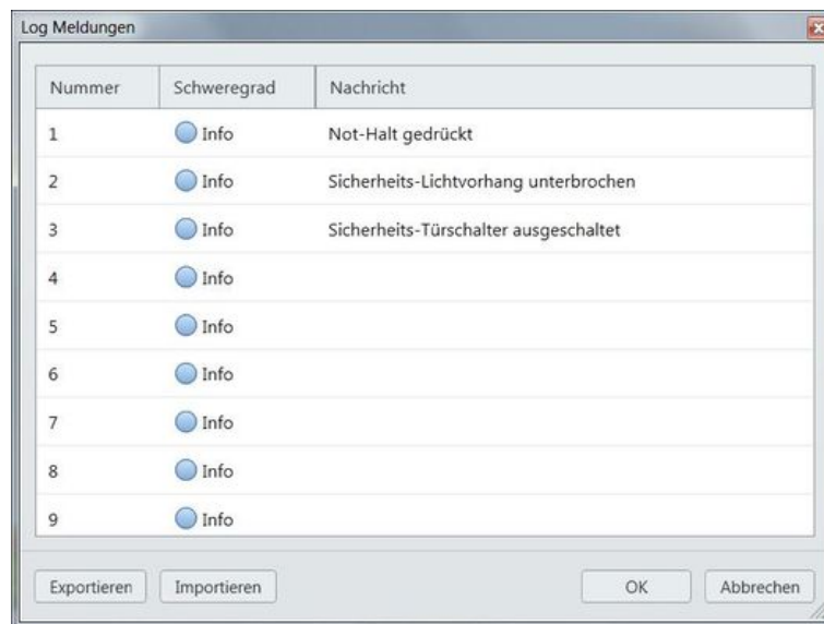
Abb. 75: Verfügbare Meldungen im Funktionsblock Log-Generator
