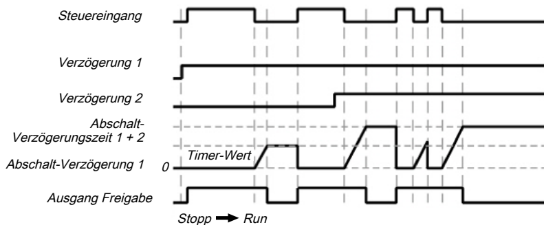
Abb. 85: Ablauf-/Timingdiagramm für den Funktionsblock Einstellbare Abschaltverzögerung mit Abschaltverzögerungszeit 1 und Abschaltverzögerungszeit 2
