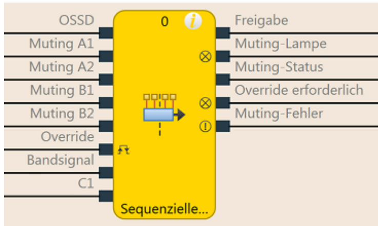
Abb. 123: Logische Anschlüsse für den Funktionsblock Sequenzielles Muting
