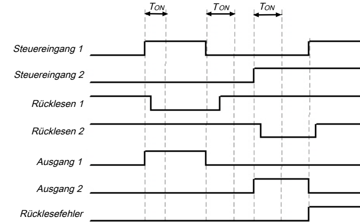
Abb. 95: Ablauf-/Timingdiagramm für Richtungsventil
