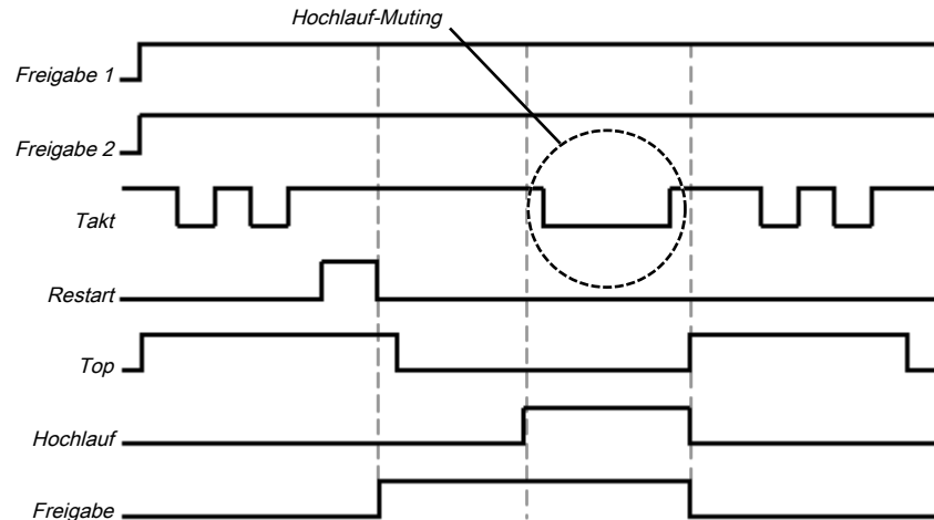
Abb. 161: Ablauf-/ Timingdiagramm für Hochlauf-Muting im Standard-Modus im Zweitaktbetrieb
