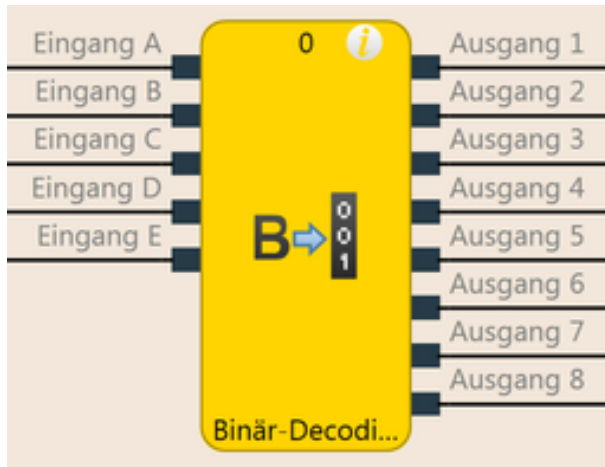
Abb. 70: Logische Anschlüsse für den Funktionsblock Binär-Decodierer
