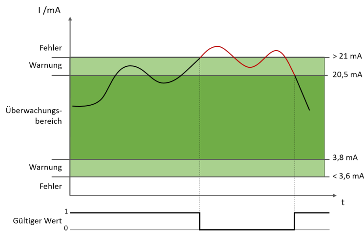
Abb. 41: Beispiel: Wert überschreitet den Überwachungsbereich (Sensor 4-20mA)
