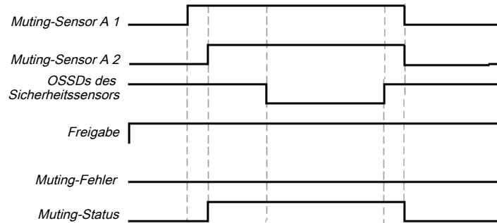
Abb. 128: Gültige Muting-Sequenz bei Benutzung der Konfigurations-Grundeinstellung
