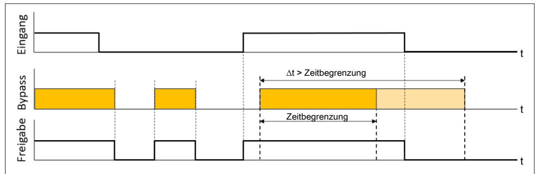
Abb. 180: Bypass-Funktion mit Zeitbegrenzung t
