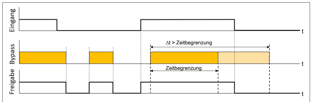
Abb. 168: Bypass-Funktion mit Zeitbegrenzung t
