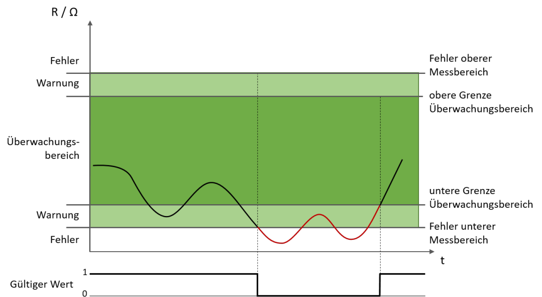
Abb. 42: Beispiel: Wert unterschreitet den Überwachungsbereich (Sensor RTD)
