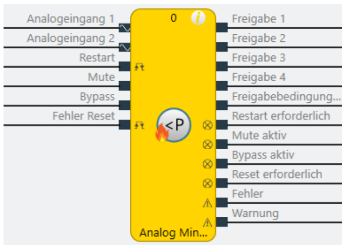
Abb. 181: Logische Anschlüsse für den Funktionsblock Analog Min Druck
