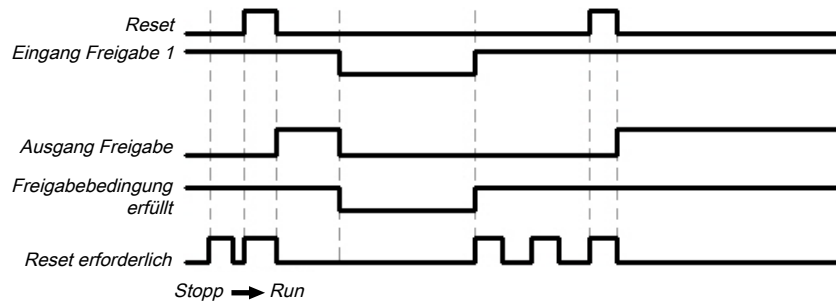
Abb. 81: Ablauf-/Timingdiagramm für den Funktionsblock Restart
