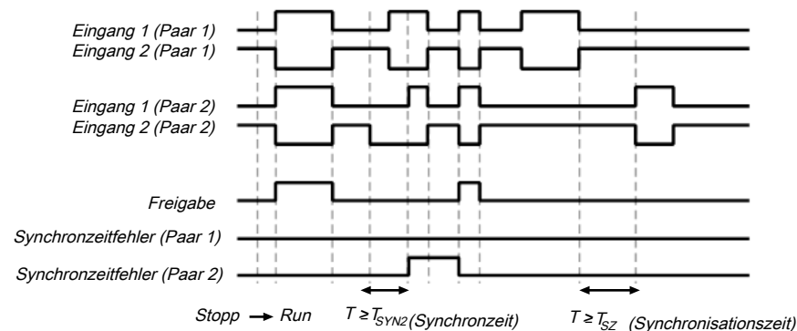
Abb. 114: Ablauf-/Timingdiagramm für den Funktionsblock Zweihand Typ IIIC
