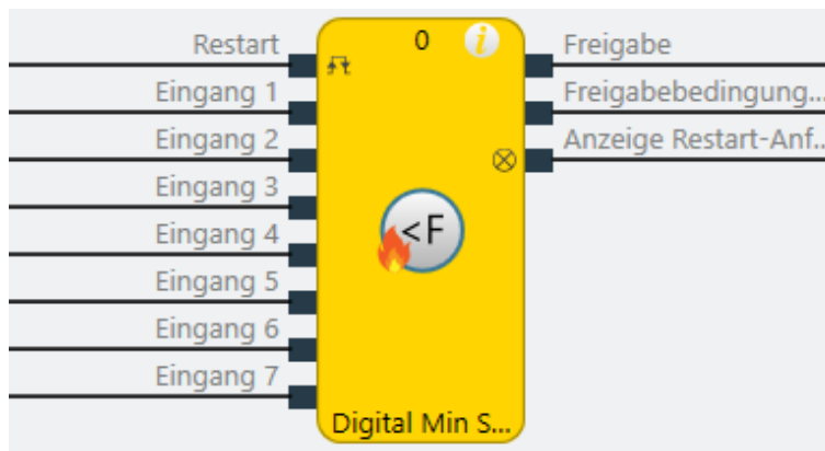
Abb. 208: Logische Anschlüsse für den Funktionsblock Digital Min Strömung
