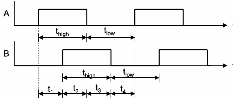
Abb. 99: Signalmuster für A/B-Pulsgeber mit 90° Phasenversatz
