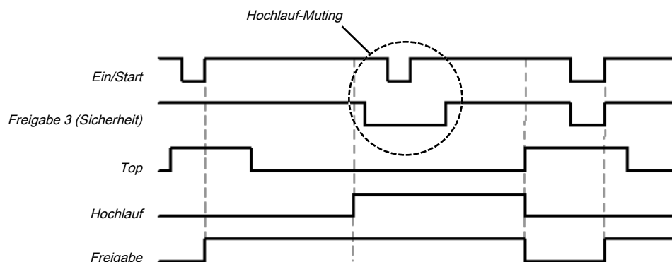
Abb. 152: Ablauf-/ Timingdiagramm für den Funktionsblock Presse Einzelhub Hochlauf-Muting von Ein/Start und Freigabe 3 (Sicherheit)
