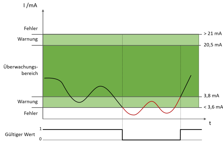
Abb. 40: Beispiel: Wert unterschreitet den Überwachungsbereich (Sensor 4-20mA)
