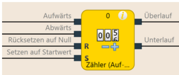
Abb. 58: Logische Anschlüsse für den Funktionsblock Zähler (Auf- und Abwärts)
