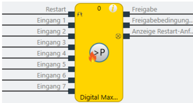
Abb. 206: Logische Anschlüsse für den Funktionsblock Digital Max Druck
