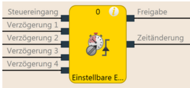
Abb. 88: Funktionsblockdiagramm für den Funktionsblock Einstellbare Einschaltverzögerung
