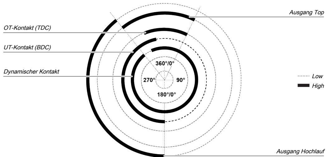
Abb. 135: Pressenzyklus für den Funktionsblock Kontaktmonitor Exzenterpresse mit Dynamischer Kontakt beim Aufwärts-hub
