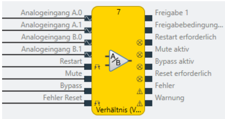
Abb. 176: Logische Anschlüsse für den Funktionsblock Verhältnis
