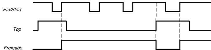
Abb. 154: Ablauf-/ Timingdiagramm für den Funktionsblock Presse Einzelhub bei Konfiguration von Ein/Start auf 2 - Einmalig Start
