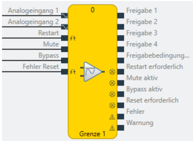
Abb. 169: Logische Anschlüsse für den Funktionsblock Grenze
