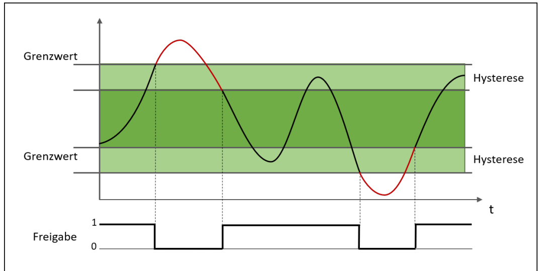
Abb. 202: Überwachung auf „Innerhalb eines Bereiches“
