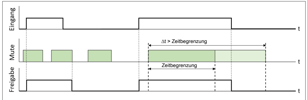
Abb. 179: Muting-Funktion mit Zeitbegrenzung t
