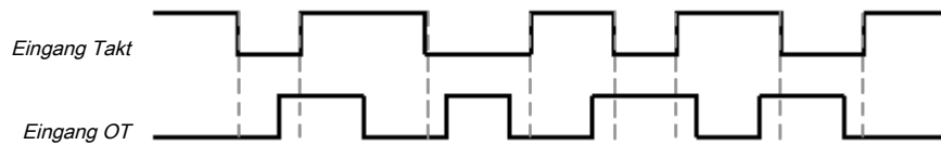
Abb. 162: Gültige Eingriffe, wenn der Parameter Start des ersten Takts auf 2 - Nach dem Start des Hochlaufs gesetzt ist.
