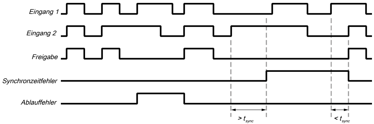
Abb. 106: Ablauf-/Timingdiagramm für den Funktionsblock Not-Halt
