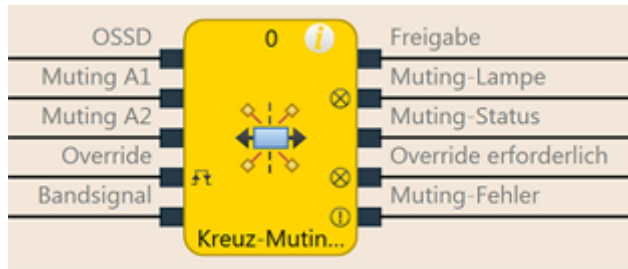
Abb. 129: Logische Anschlüsse für den Funktionsblock Kreuz-Muting (zweiseitig)
