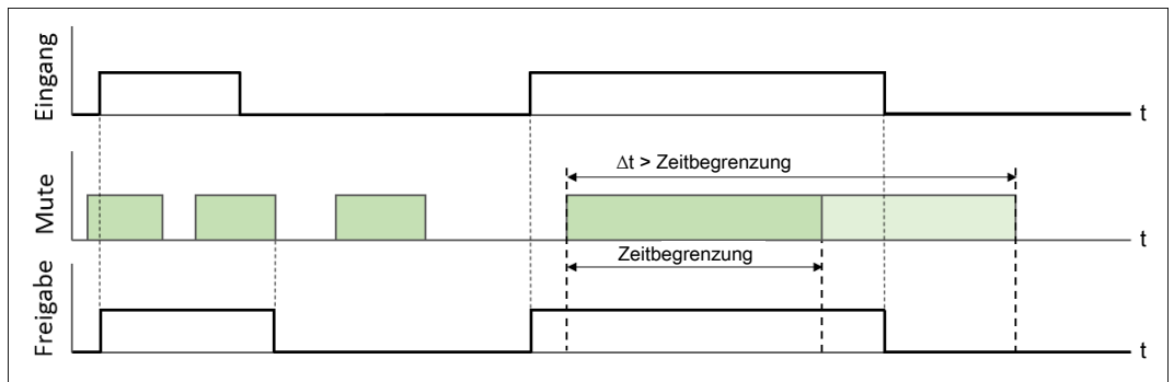
Abb. 167: Muting-Funktion mit Zeitbegrenzung t
