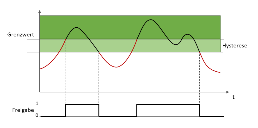
Abb. 192: Überwachung auf "Unterschreitung"
