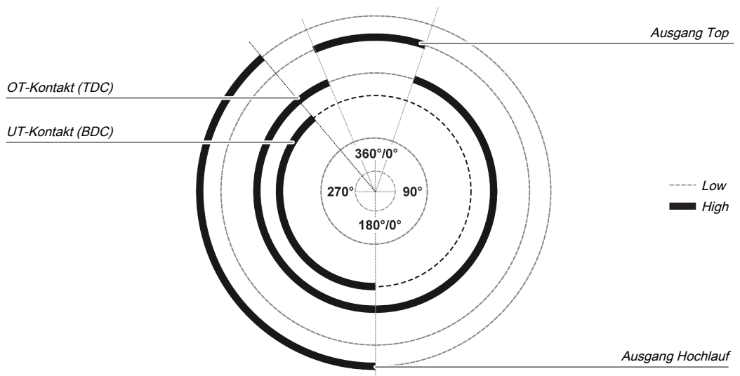
Abb. 142: Pressenzyklus für den Funktionsblock Kontaktmonitor Universalpresse mit fallender Flanke von UT-Kontakt (BDC) vor OT-Kontakt (TDC)
