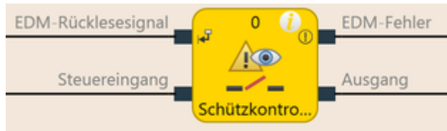
Abb. 90: Funktionsblockdiagramm für den Funktionsblock EDM
