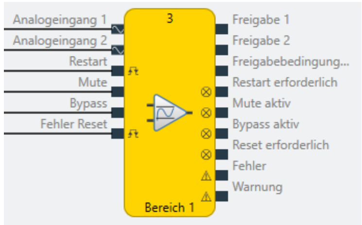
Abb. 172: Logische Anschlüsse für den Funktionsblock Bereich
