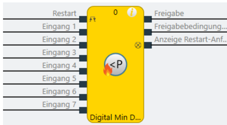
Abb. 204: Logische Anschlüsse für den Funktionsblock Digital Min Druck
