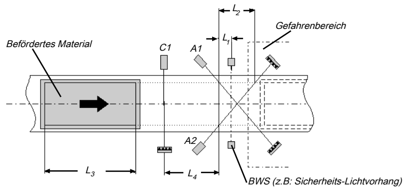
Abb. 127: Beispiel für Kreuz-Muting (einseitig) mit Eingang C1
