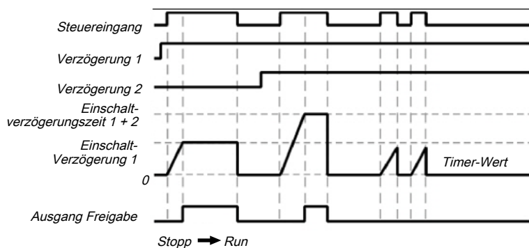
Abb. 89: Ablauf-/Timingdiagramm für den Funktionsblock Einstellbare Einschaltverzögerung mit Einschaltverzögerungszeit 1 und Einschaltverzögerungszeit 2
