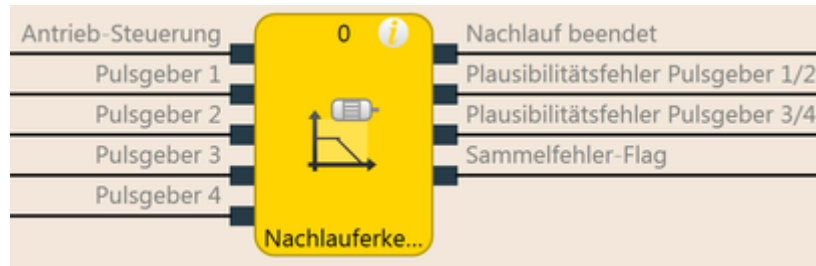
Abb. 98: Logische Anschlüsse für den Funktionsblock Nachlauferkennung
