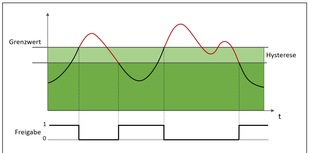
Abb. 170: Überwachung auf "Überschreitung"
