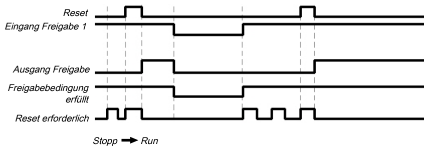
Abb. 209: Ablauf-/Timing-Diagramm für den Funktionsblock
