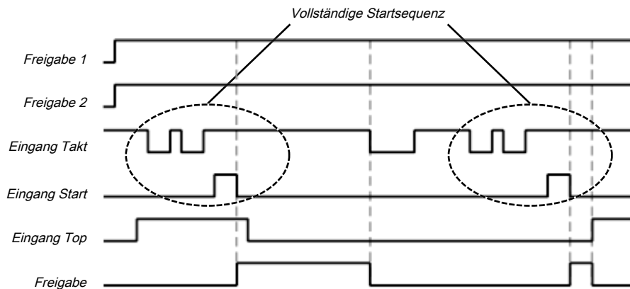
Abb. 163: Ablauf-/ Timingdiagramm, wenn der Eingang Takt Low, Hochlauf-Muting inaktiv und Wiederanlaufsperr auf 2 - immer gesetzt ist.
