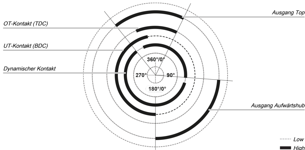
Abb. 136: Pressenzyklus für den Funktionsblock Kontaktmonitor Exzenterpresse mit Dynamischer Kontakt beim Hochlauf und bei der Abwärtsbewegung
