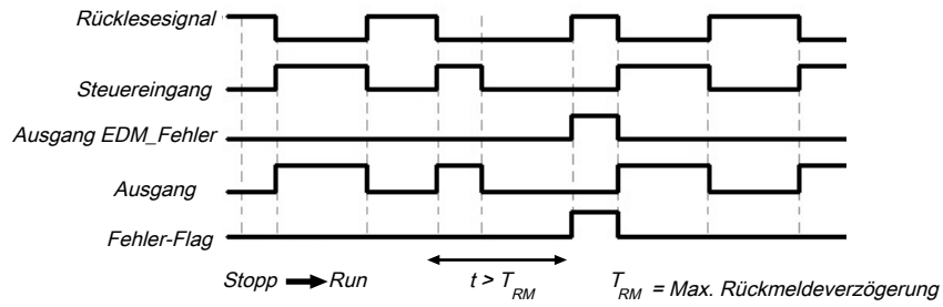
Abb. 91: Ablauf-/Timingdiagramm für den Funktionsblock EDM
