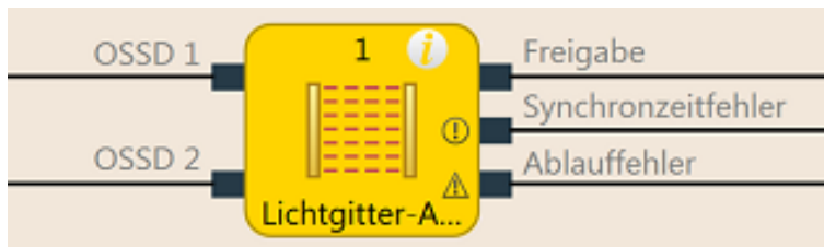
Abb. 108: Funktionsblockdiagramm für den Funktionsblock Lichtgitter-Auswertung
