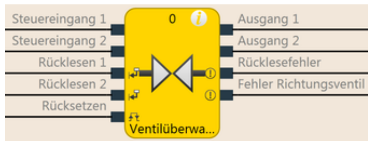
Abb. 92: Logische Anschlüsse für den Funktionsblock Ventilüberwachung, konfiguriert für ein Richtungsventil
