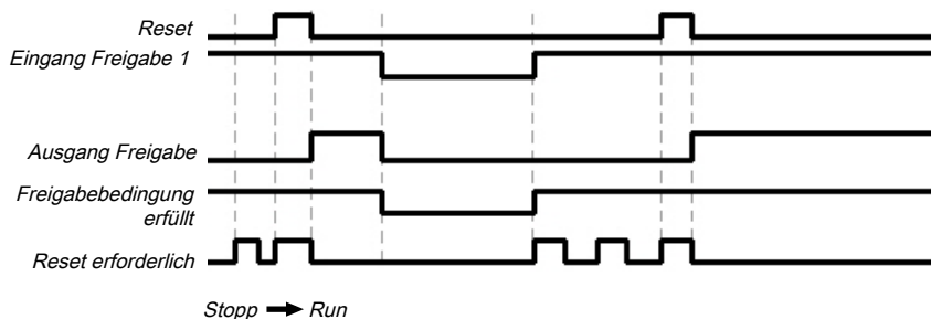
Abb. 211: Ablauf-/Timing-Diagramm für den Funktionsblock
