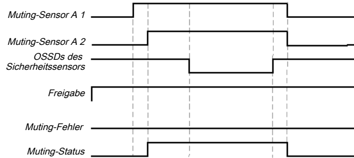
Abb. 131: Gültige Muting-Sequenz bei Benutzung der Konfigurations-Grundeinstellung
