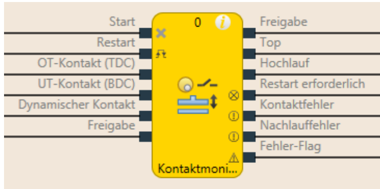
Abb. 132: Logische Anschlüsse für den Funktionsblock Kontaktmonitor Exzenterpresse
