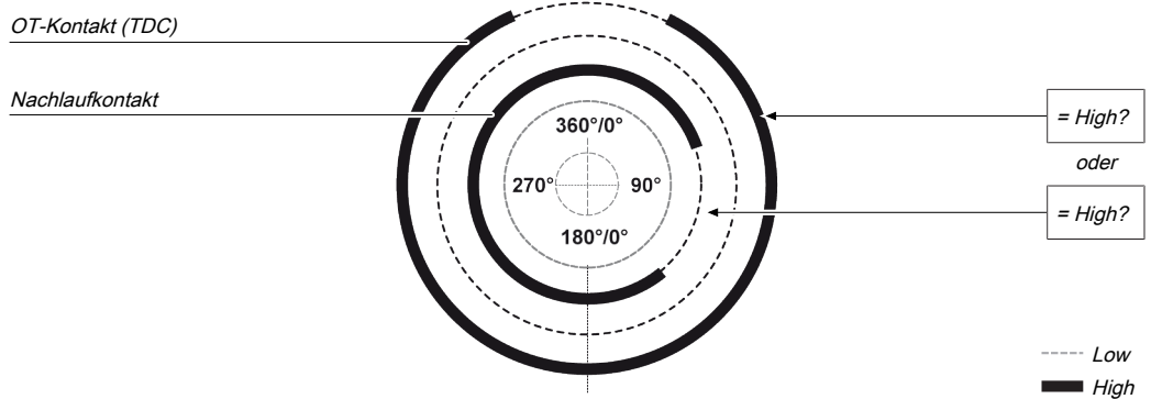
Abb. 139: Kontaktüberwachung mit dem Funktionsblock Kontaktmonitor Universalpresse mit aktiviertem Nachlauf
