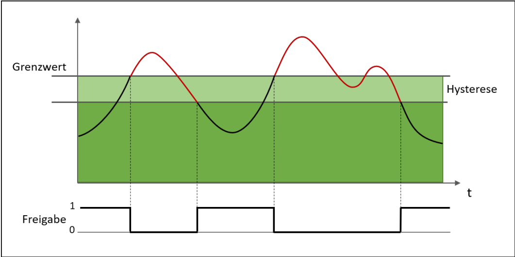
Abb. 182: Überwachung auf "Überschreitung"
