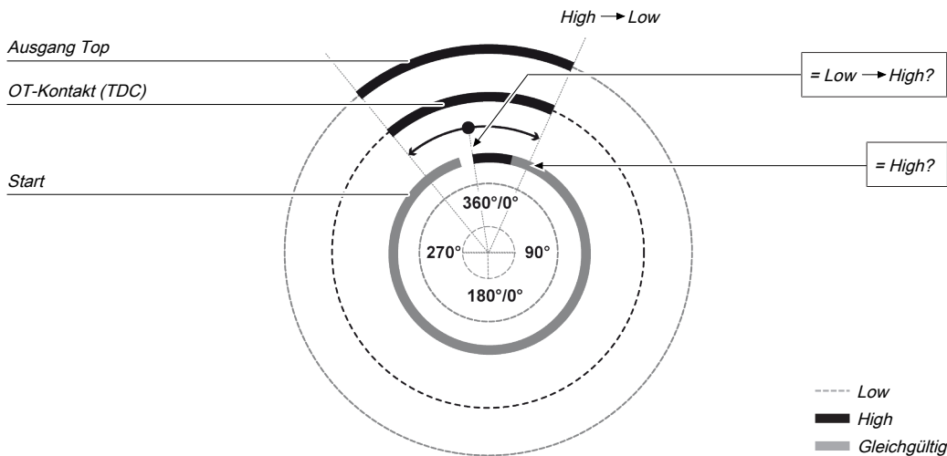
Abb. 134: Nachlaufüberwachung mit dem Funktionsblock Kontaktmonitor Exzenterpresse
