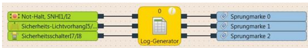
Abb. 73: Konfigurationsbeispiel für Log-Generator mit zwei Not-Halt-Tastern und einem Sicherheits-Schalter
