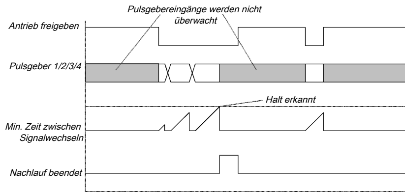
Abb. 103: Ablauf-/Timingdiagramm für den Funktionsblock 'Nachlauferkennung'
