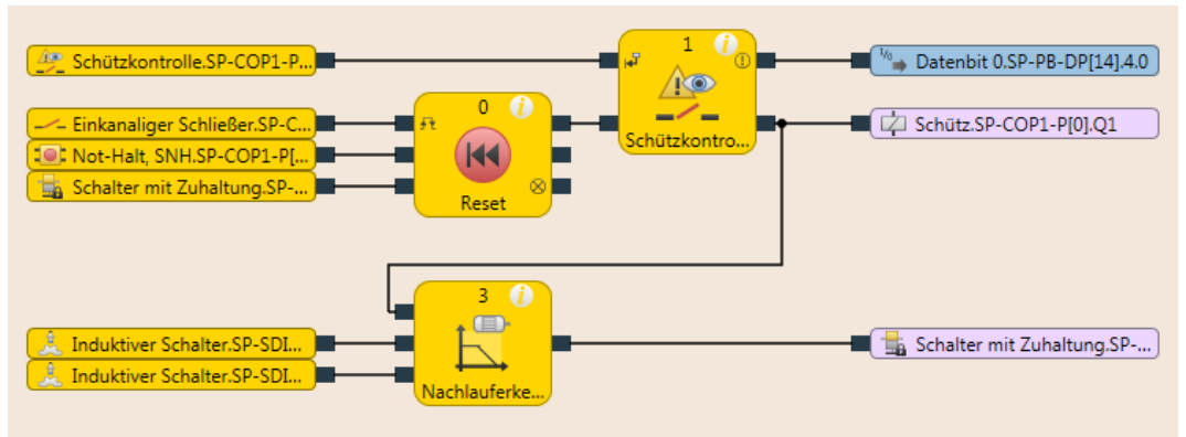
Abb. 102: Logikbeispiel für den Funktionsblock 'Nachlauferkennung'
