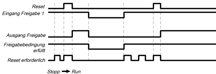
Abb. 215: Ablauf-/Timing-Diagramm für den Funktionsblock
