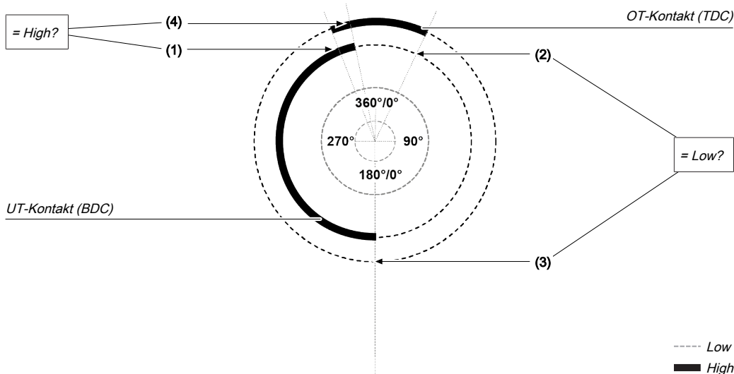
Abb. 133: Kontaktüberwachung mit dem Funktionsblock Kontaktmonitor Exzenterpresse
