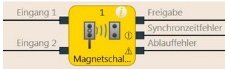
Abb. 107: Logische Anschlüsse für den Funktionsblock Magnetschalter
