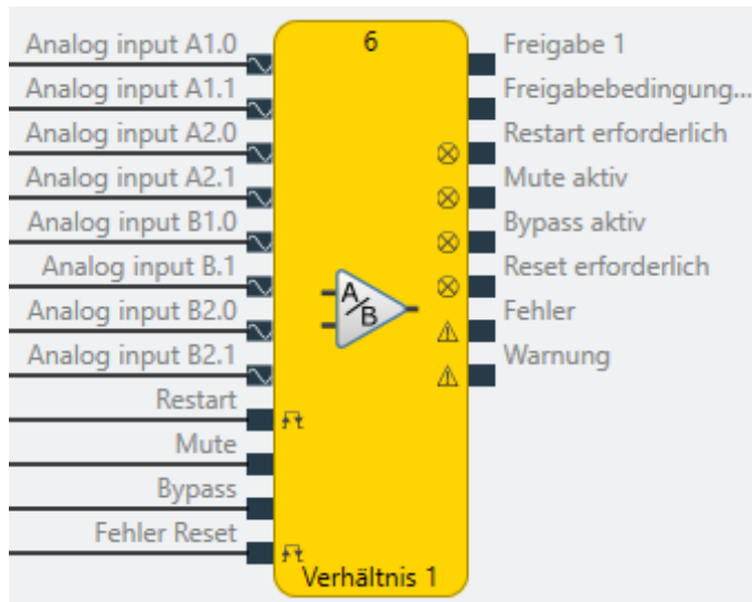
Abb. 174: Logische Anschlüsse für den Funktionsblock Verhältnis
