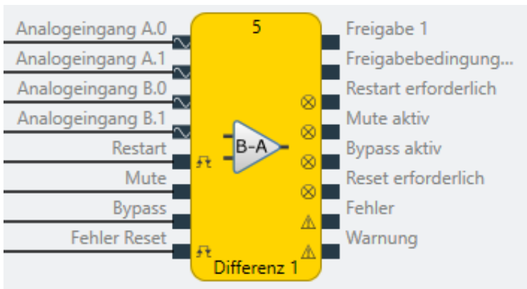
Abb. 175: Logische Anschlüsse für den Funktionsblock Differenz
