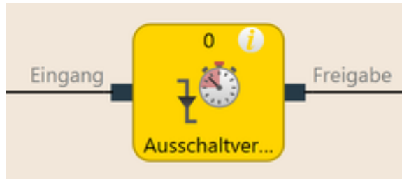
Abb. 82: Funktionsblockdiagramm für den Funktionsblock Abschaltverzögerung
