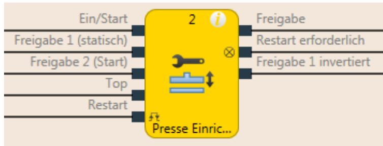
Abb. 147: Logische Anschlüsse für den Funktionsblock Presse Einrichten
