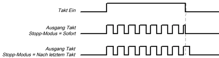
Abb. 57: Timingdiagramm für den Funktionsblock Taktgenerator
