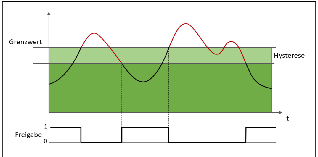
Abb. 194: Überwachung auf "Überschreitung"
