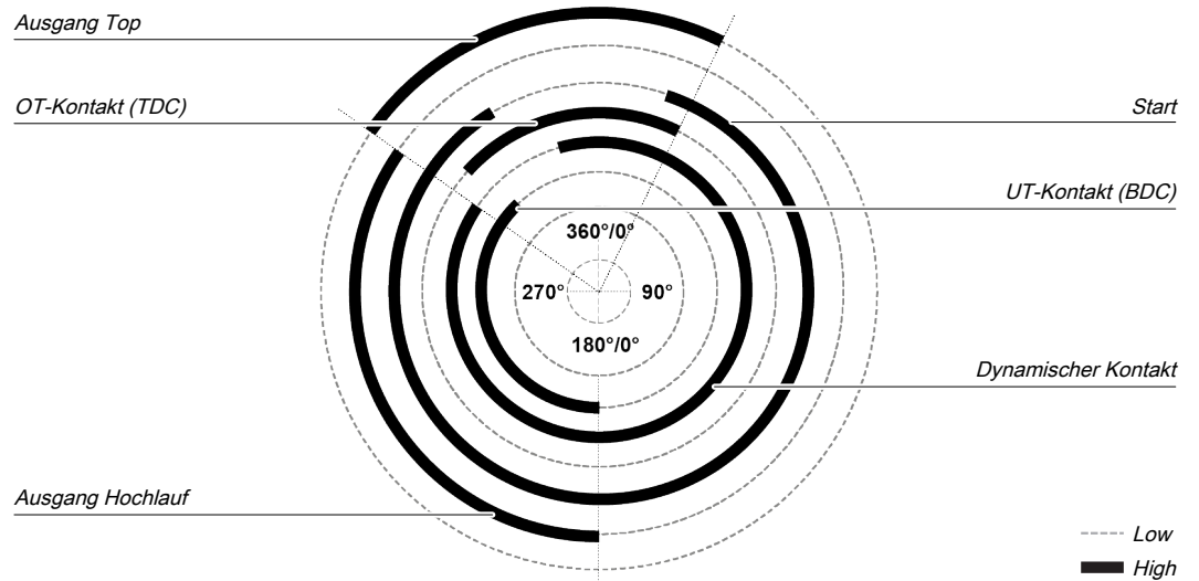
Abb. 146: Kontakt- und Ausgangsfolge einer Universalpresse bei einem fehlerfreien Ablauf (Beispiel)
