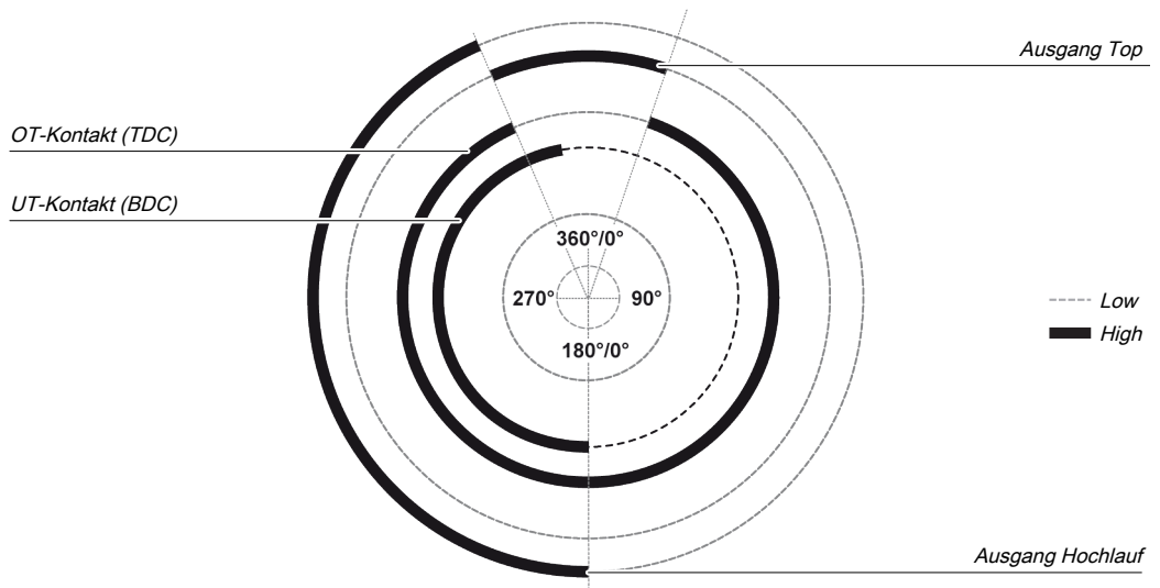
Abb. 141: Pressenzyklus für den Funktionsblock Kontaktmonitor Universalpresse mit fallender Flanke von OT-Kontakt (TDC) vor UT-Kontakt (BDC)
