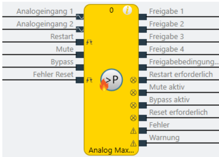
Abb. 184: Logische Anschlüsse für den Funktionsblock Analog Max Druck
