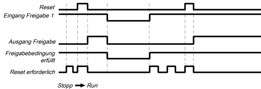
Abb. 207: Ablauf-/Timing-Diagramm für den Funktionsblock
