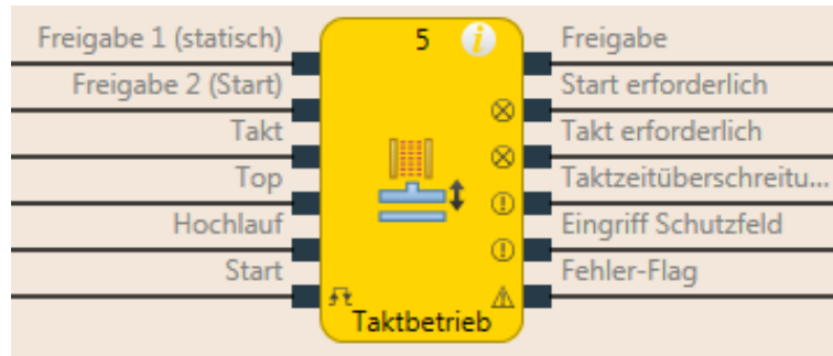
Abb. 157: Logische Anschlüsse für den Funktionsblock Taktbetrieb
