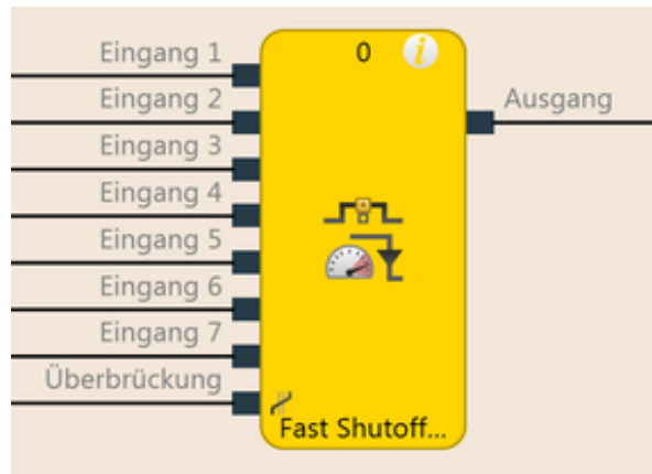
Abb. 60: Logische Anschlüsse für den Funktionsblock Fast Shut Off mit Bypass
