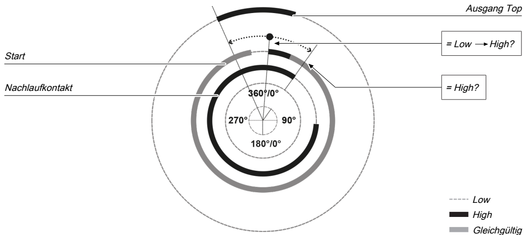
Abb. 144: Nachlaufüberwachung mit dem Funktionsblock Kontaktmonitor Universalpresse
