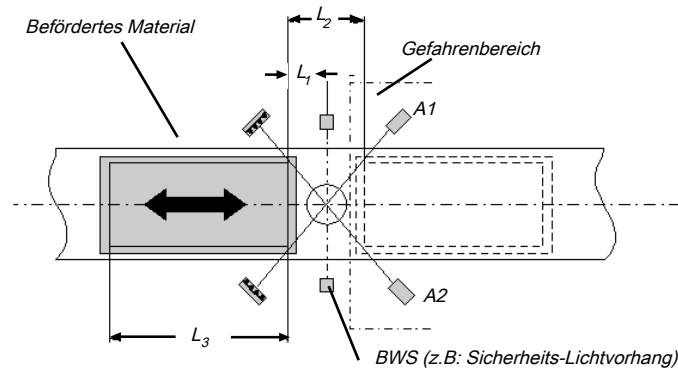
Abb. 130: Kreuz-Muting (zweiseitig) mit bidirektionaler Bewegung von Material
