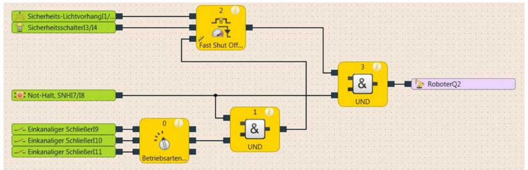
Abb. 66: Beispiel für Fast Shut Off mit Bypass mit mehr als einer Bedingung für Bypass
