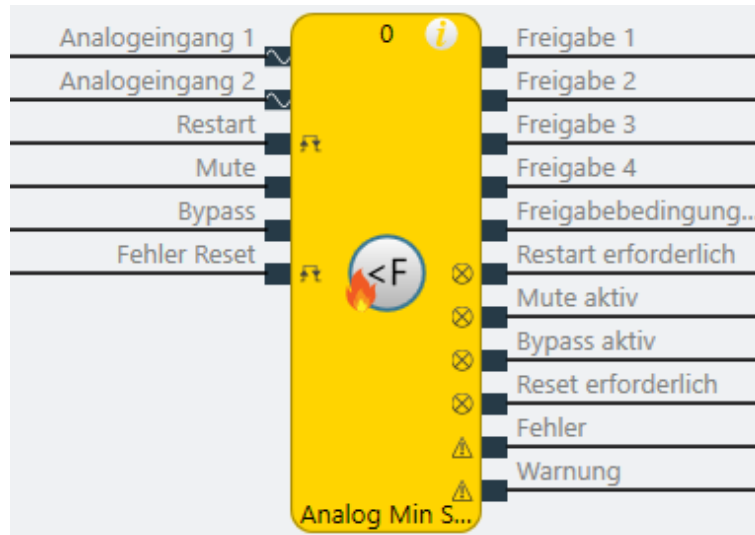
Abb. 187: Logische Anschlüsse für den Funktionsblock Analog Min Strömung
