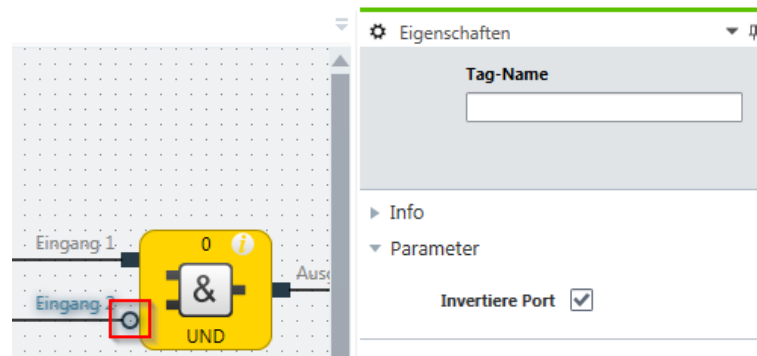
Abb. 46: Beispiel eines UND-Funktionsblocks mit einem invertierten Eingang
