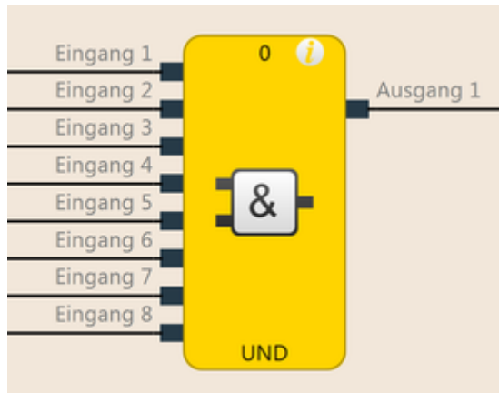
Abb. 49: Funktionsblockdiagramm für den Funktionsblock UND
