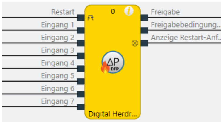
Abb. 218: Logische Anschlüsse für den Funktionsblock Herdraumdruck
