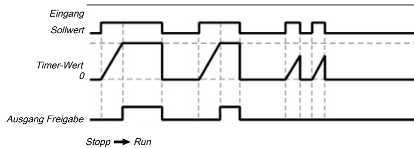
Abb. 87: Ablauf-/Timingdiagramm für den Funktionsblock Einschaltverzögerung
