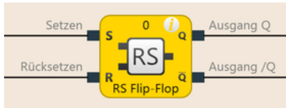
Abb. 53: Logische Anschlüsse für den Funktionsblock RS Flip-Flop
