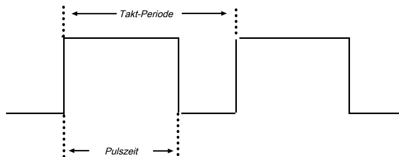
Abb. 56: Parameterdiagramm für den Funktionsblock „Taktgenerator“
