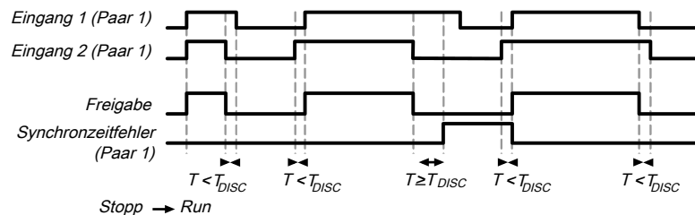
Abb. 111: Ablauf-/Timingdiagramm für Funktionsblock Schalter-Auswertung, Kategorie 4, zweikanalig ohne Funktionstest
