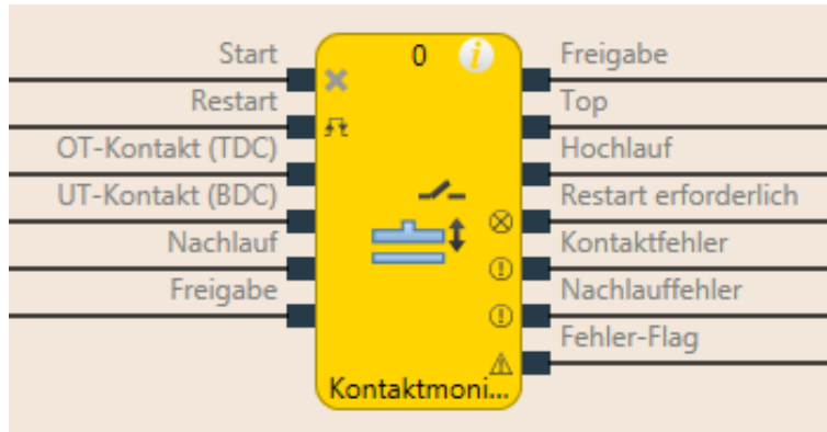
Abb. 138: Logische Anschlüsse für den Funktionsblock Kontaktmonitor Universalpresse
