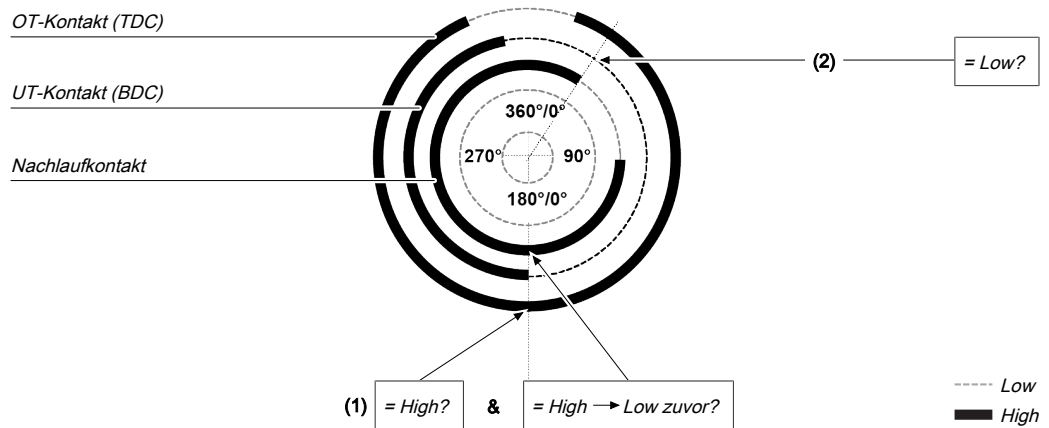
Abb. 145: Kontaktüberwachung mit dem Funktionsblock Kontaktmonitor Universalpresse mit aktiviertem UT-Kontakt (BDC) und Nachlauf
