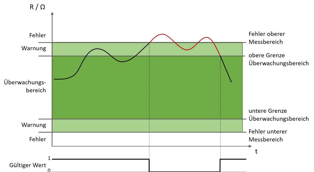
Abb. 43: Beispiel: Wert überschreitet den Überwachungsbereich (Sensor RTD)
