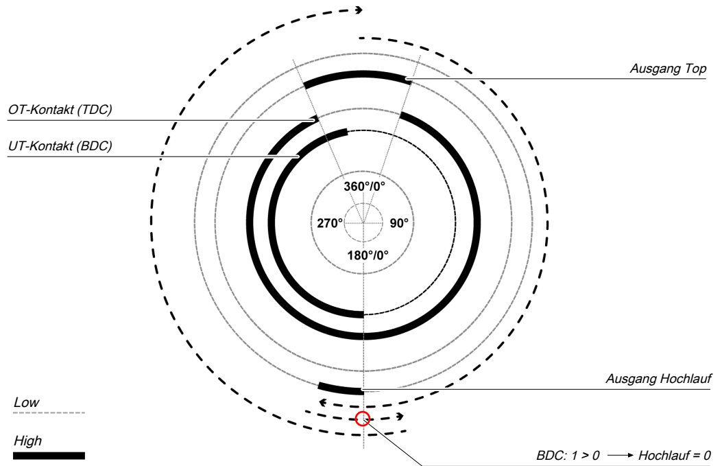
Abb. 143: Pressenzyklus für den Funktionsblock Kontaktmonitor Universalpresse mit 2 BDC-Übergängen
