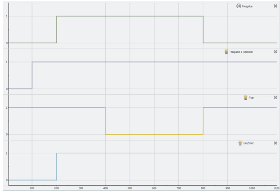
Abb. 151: Minimalistischer Ablauf Baustein Presse Einrichten
