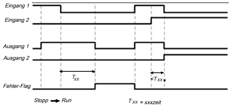
Abb. 97: Ablauf-/Timingdiagramm für den Funktionsblock Betriebsartenwahlschalter
