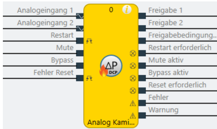
Abb. 199: Logische Anschlüsse für den Funktionsblock Analog Kaminzug
