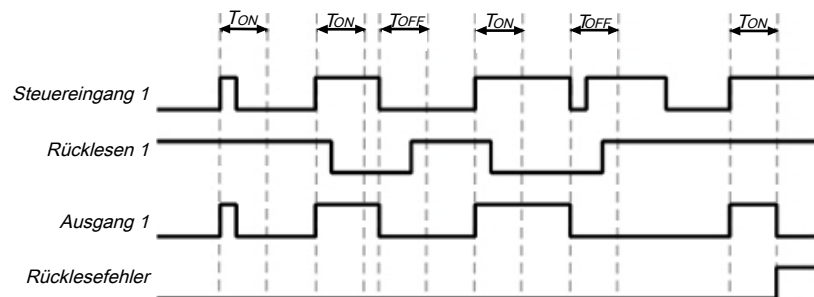
Abb. 93: Ablauf-/Timingdiagramm für Einzelventil im manuellen Resetmodus
