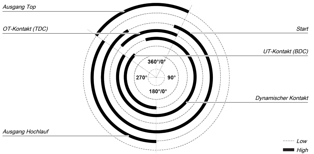
Abb. 137: Kontakt- und Ausgangsfolge einer Exzenterpresse bei einem fehlerfreien Ablauf (Beispiel)
