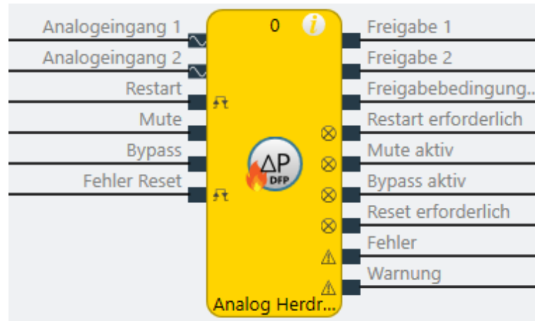
Abb. 201: Logische Anschlüsse für den Funktionsblock Analog Herdraumdruck
