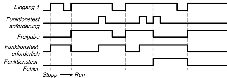
Abb. 110: Ablauf-/Timingdiagramm für Funktionsblock Schalter-Auswertung, Kategorie 2, einkanalig mit Funktionstest
