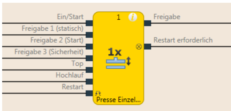
Abb. 150: Logische Anschlüsse für den Funktionsblock Presse Einzelhub
