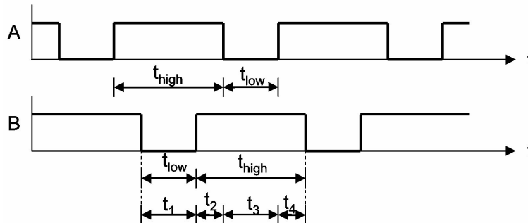
Abb. 100: Signalmuster für 1/3-Lücken-Pulsgeber mit 180° Phasenversatz
