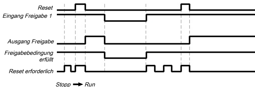
Abb. 79: Ablauf-/Timingdiagramm für den Funktionsblock Reset
