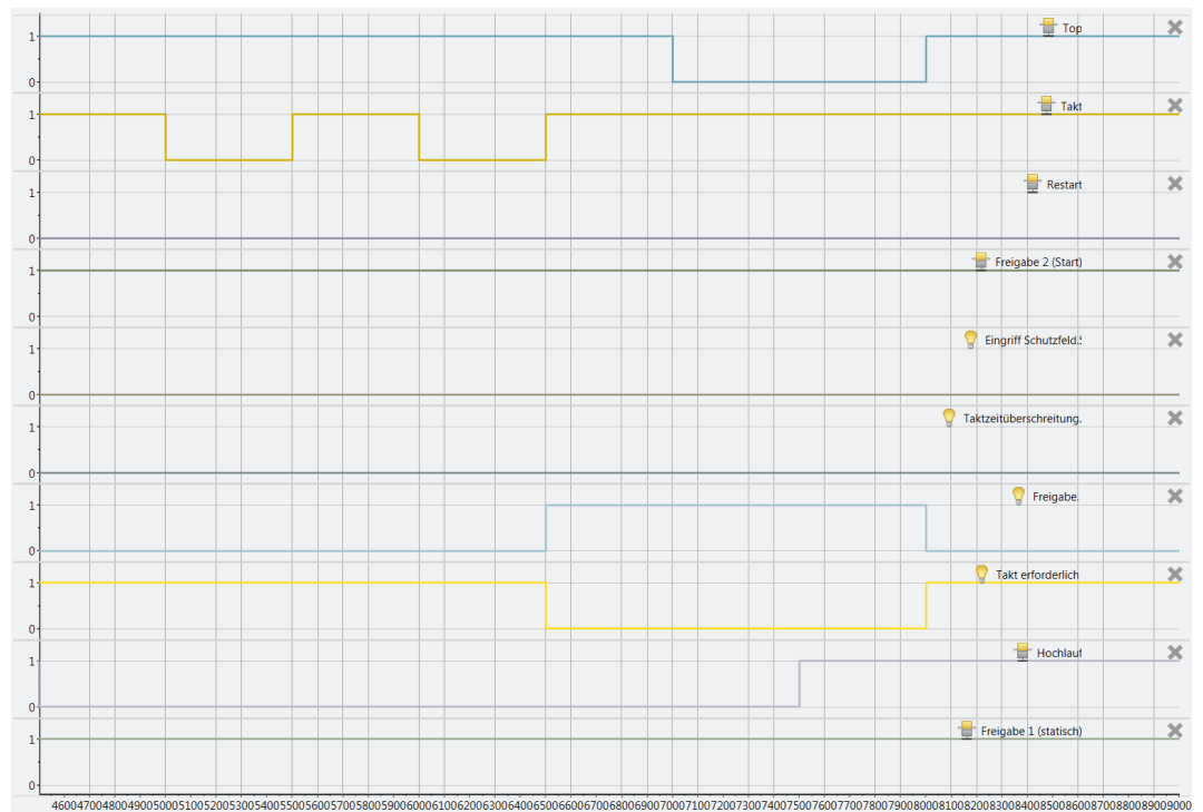
Abb. 158: Ablauf-/ Timingdiagramm für eine vollständige Sequenz im Standard-Mode mit 2 parametrieren Eingriffen ohne Wiederanlaufsperr
