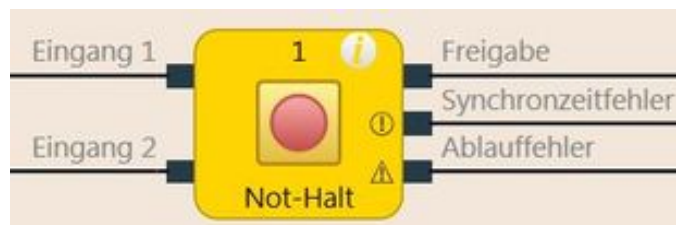
Abb. 105: Funktionsblockdiagramm für den Funktionsblock Not-Halt
