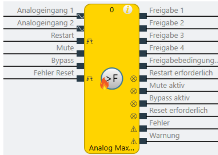
Abb. 190: Logische Anschlüsse für den Funktionsblock Analog Max Strömung
