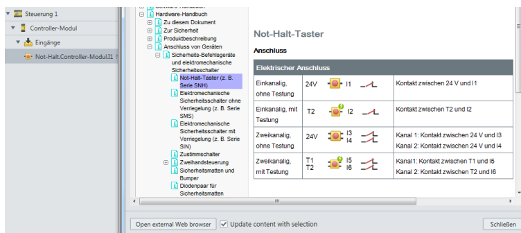
Abb. 10: Programmhilfe zum gewählten Objekt "Not-Halt-Taster"
