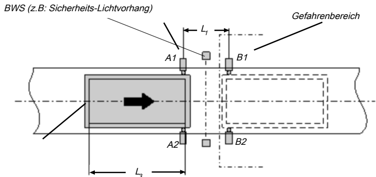
Abb. 121: Muting mit zwei parallelen Sensorpaaren
