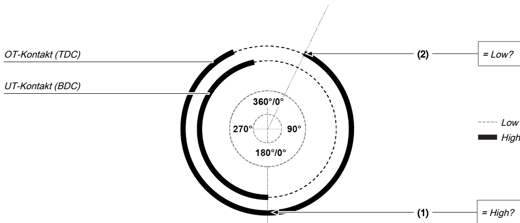
Abb. 140: Kontaktüberwachung mit dem Funktionsblock Kontaktmonitor Universalpresse mit aktiviertem UT-Kontakt (BDC)
