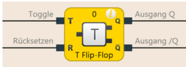
Abb. 52: Funktionsblockdiagramm für den Funktionsblock T-Flip-Flop
