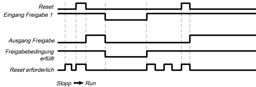
Abb. 213: Ablauf-/Timing-Diagramm für den Funktionsblock
