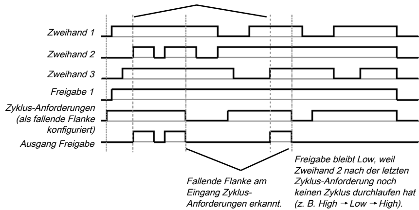
Abb. 116: Ablauf-/Timingdiagramm für den Funktionsblock Mehrfach-Zweihand
