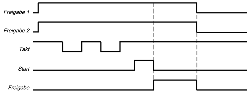
Abb. 159: Ablauf-/ Timingdiagramm für eine vollständige Startsequenz im Standard-Modus im Zweitaktbetrieb
