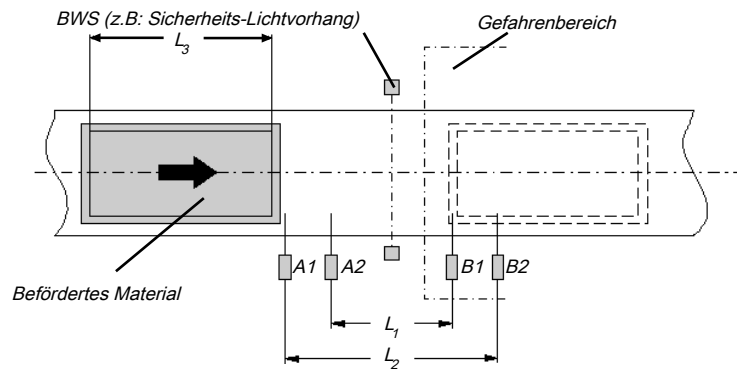
Abb. 124: Beispiel für die sequenzielle Anordnung von Muting-Sensoren
