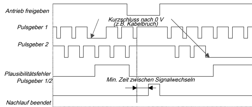
Abb. 104: Ablauf-/Timingdiagramm für den Funktionsblock 'Nachlauferkennung mit Plausibilitätsprüfung'
