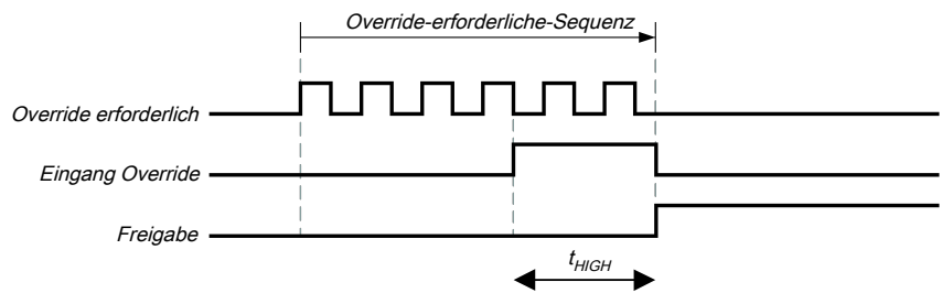
Abb. 119: Logikdiagramm für Override und Override-Anforderung]
