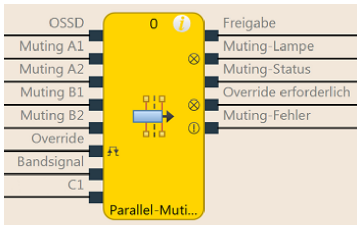
Abb. 120: Logische Anschlüsse für den Funktionsblock Parallel-Muting
