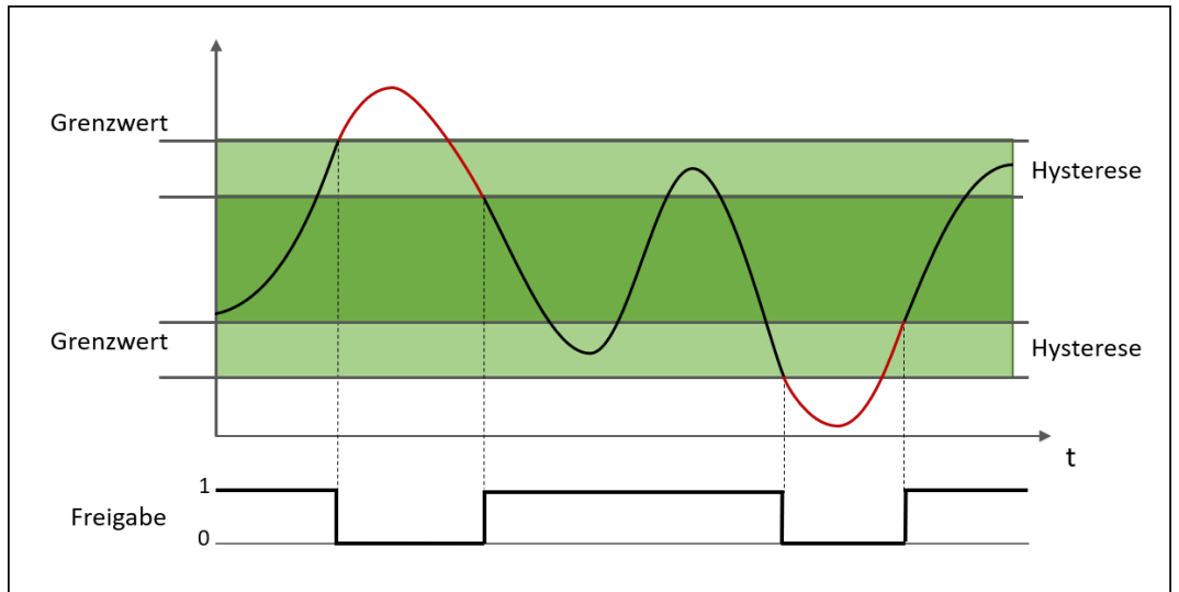
Abb. 200: Überwachung auf „Innerhalb eines Bereiches“
