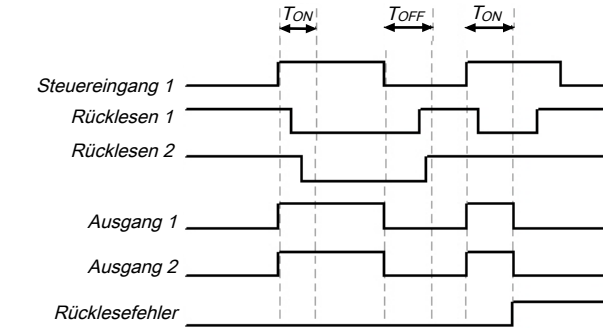
Abb. 94: Ablauf-/Timingdiagramm für Doppelventil im manuellen Resetmodus
