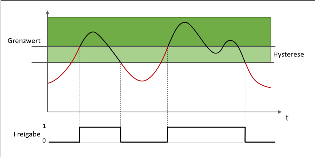
Abb. 183: Überwachung auf "Unterschreitung"
